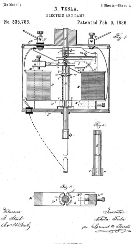
Слика 2 - Теслини први амерички патенти US 335,786 А
