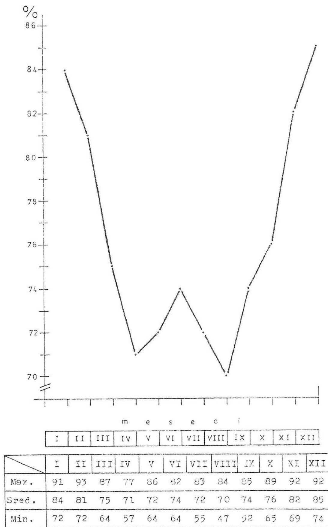
Graf.2.: Prosečne vrednosti relativne vlažnosti vazduha (1950-89)
